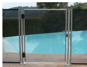
Πόρτα με αυτόματο κλείσιμο. Άνοιγμα πάντα προς τα έξω & κλείδωμα πάντα προς την πισίνα. Automatic self closing gate. Always opens towards the outside & locks towards the pool.
